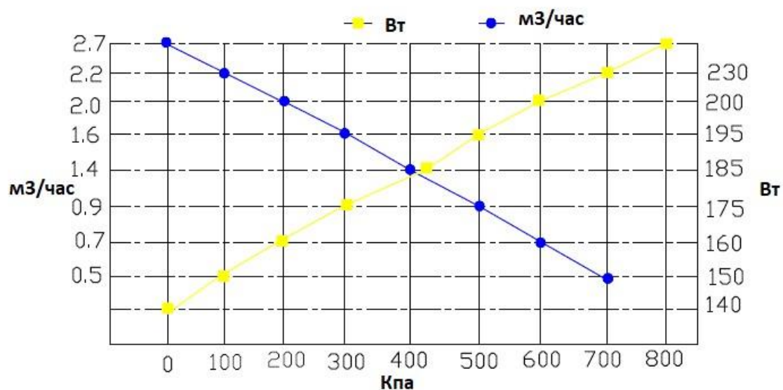
График производительности и мощности в зависимости от противодавления.
