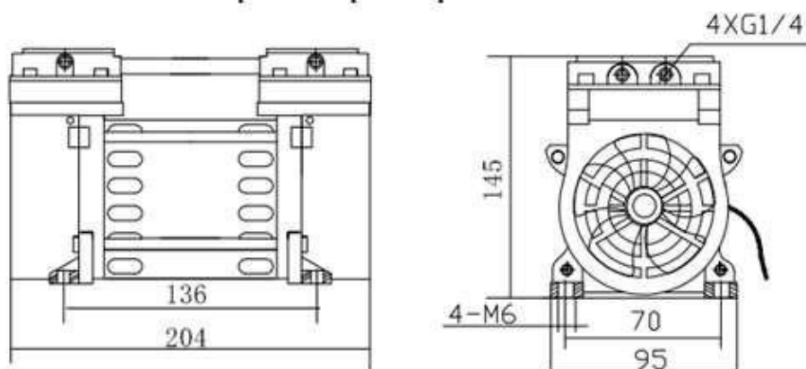
Габаритные размеры
